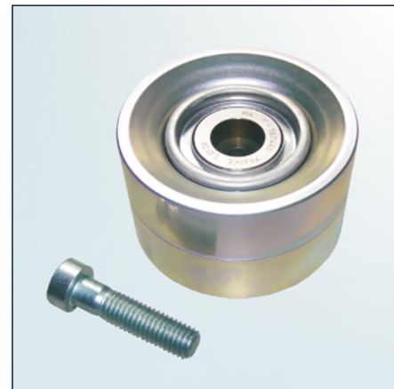
Image 2 : 532 0410 20 - nouvelle version
