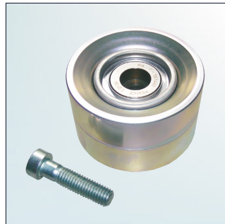
Bild 2: 532 0410 20 – nytt utförande
