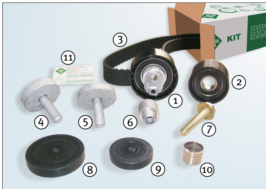
Imaginea 1 – Kit cureaua distribuție 530 0363 10
