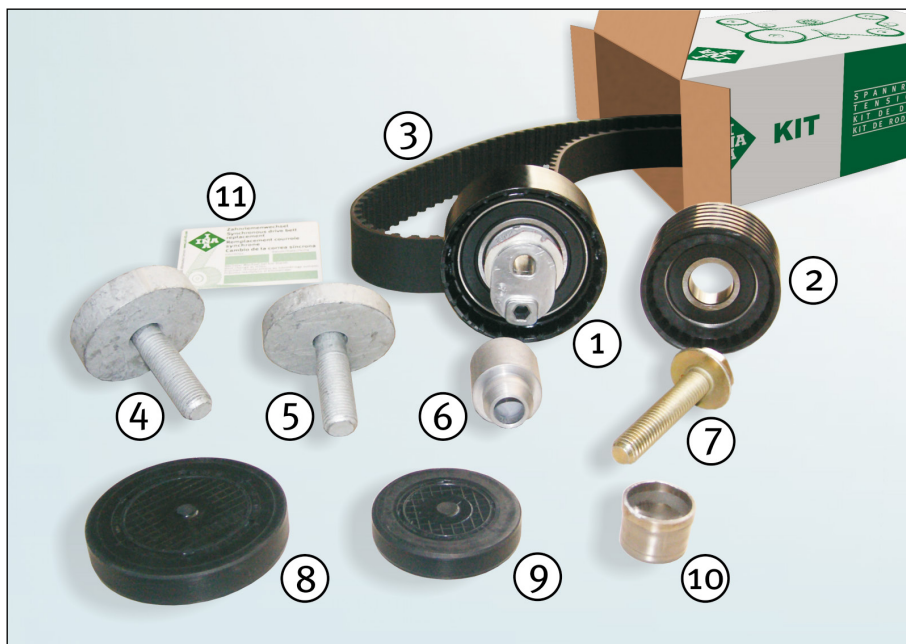
Bild 1: komplett innehåll i kuggremsatsen - INA KIT 530 0363 10
