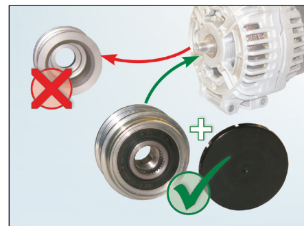
2. ábra: Generátor-szabadonfutó cseréje
