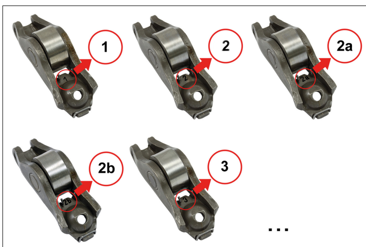
Figure 2: Exemplu de marcaje pe unele culbutoare cu contact rulant
