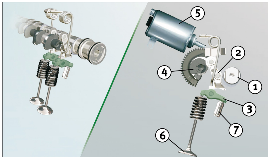
Снимка 1: Общ преглед на системата BMW Valvetronic/Подобен изглед на компонентите на системата.
