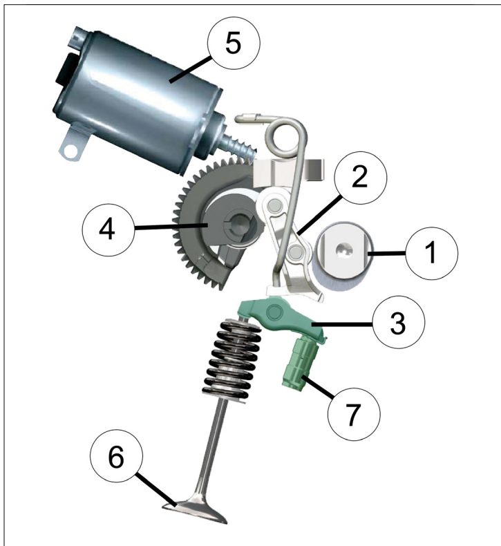
Obrázek 3: Detailní pohled na komponenty systému v BMW Valvetronic
