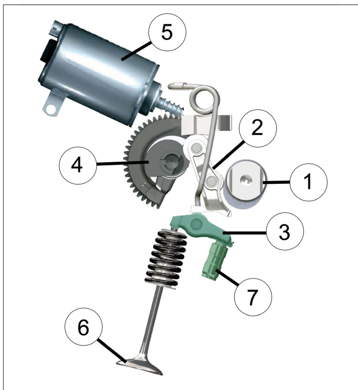
Εικόνα 3: Λεπτομερής προβολή των εξαρτημάτων του συστήματος σε ένα BMW Valvetronic
