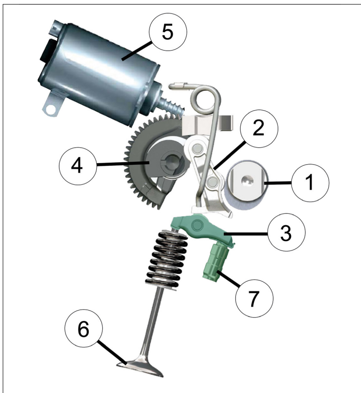
Bild 3: Detaljvy över komponenter i systemet BMW Valvetronic
