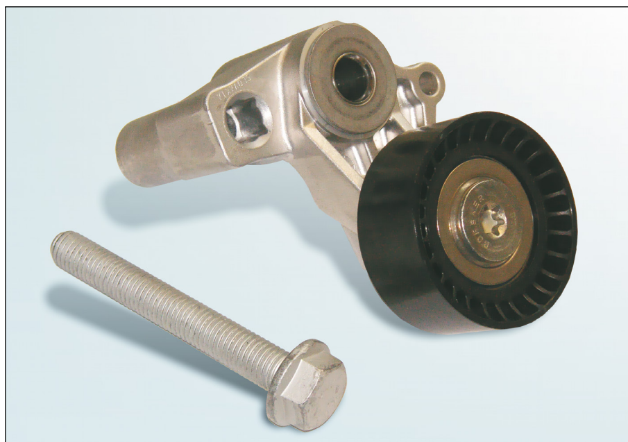
Снимка 1: 534 0100 20 – настояща конструкция
