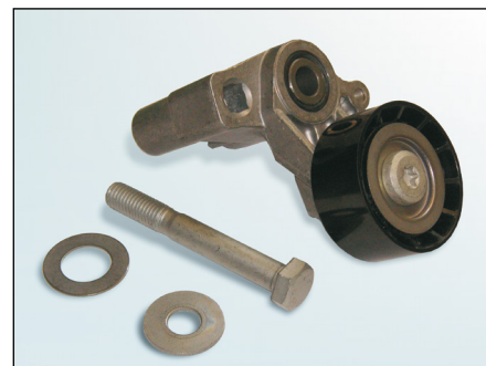
Снимка 2: 534 0100 20 – предишна конструкция
