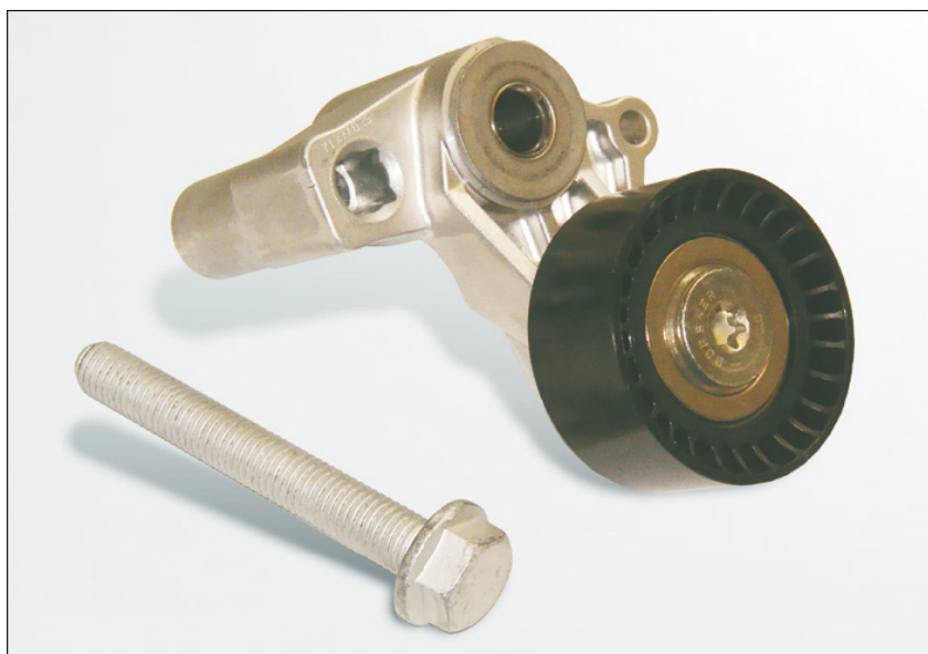
Рис. 1: 534 0100 20 – текущая конструкция
