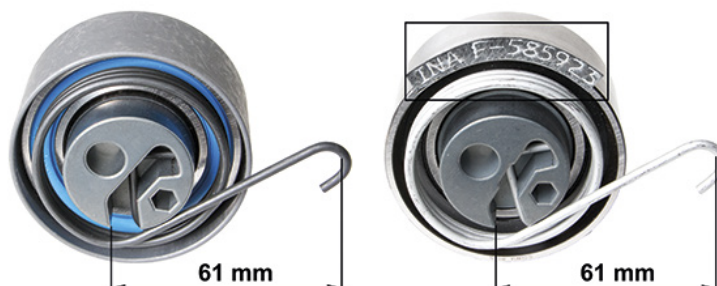
Снимка 1: 531 0535 20 – стара конструкция (отляво), нова конструкция (отдясно)
