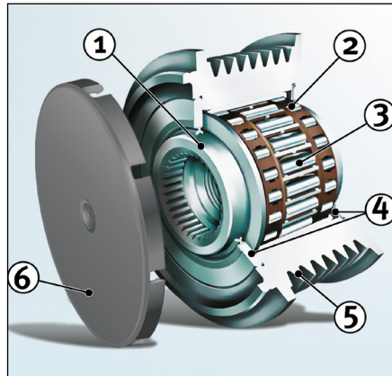
Εικόνα 4: Τροχαλία ελεύθερης περιστροφής
