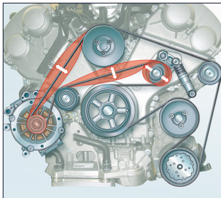
Εικόνα 1: Παράδειγμα συστήματος μετάδοσης κίνησης των συγκροτημάτων - παρουσία των κραδασμών που προκαλούνται από τη χρήση μίας συνηθισμένης άκαμπτης τροχαλίας ιμάντα στη γεννήτρια
