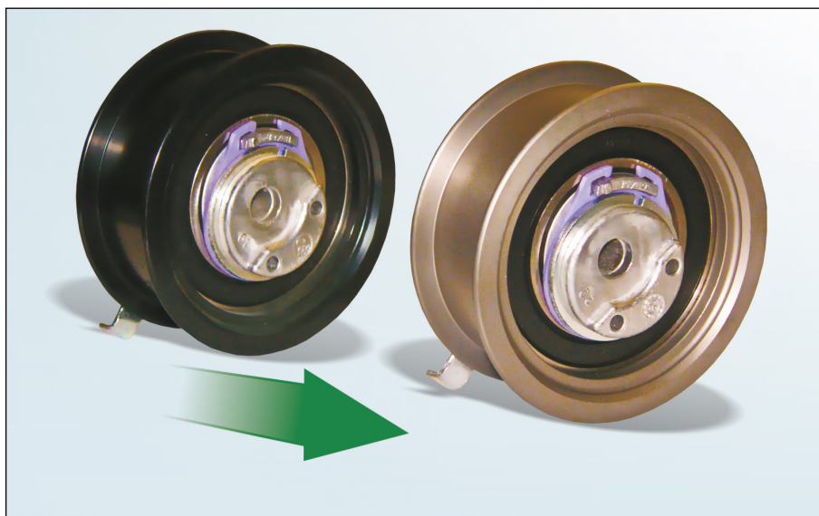
Obrázek 1: Vylepšená povrchová úprava oběžné dráhy – zde znázorněno jako příklad u objednáčného č. 531 0524 30
