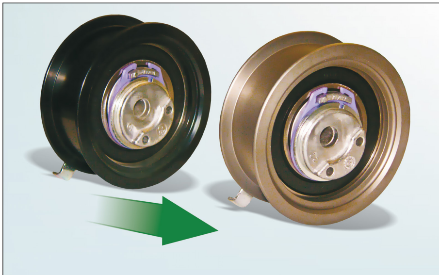
1. ábra: A futópálya javított bevonata - itt példaszerűen ábrázolták az 531 0524 30 cikkszámún
