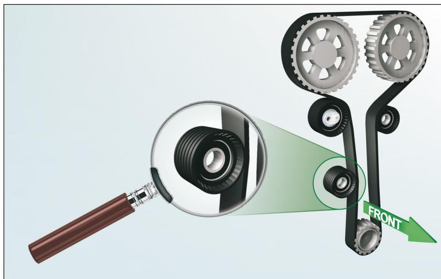
Imagine 1: Cursa curelei și poziția rolor în motorul F4R
