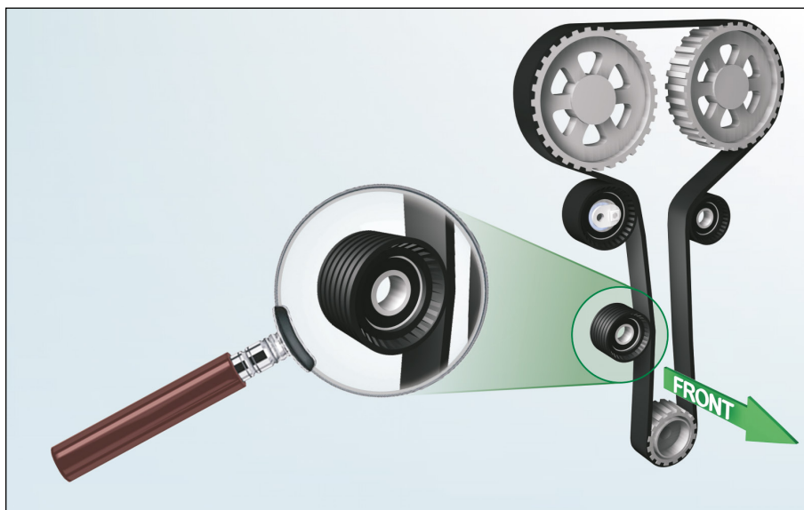
Obrázek 1: Průběh řemenu a pozice kladek v motoru F4R
