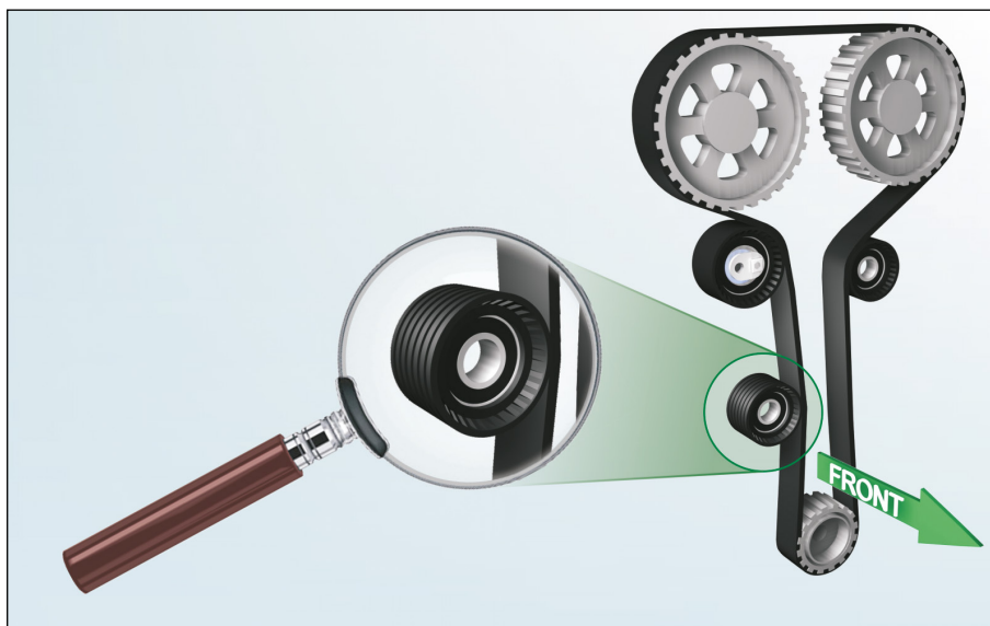
Figur 1: Remmens forløb og rullepositioner i F4R-motoren
