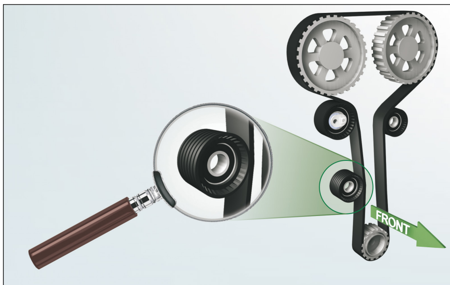
Εικόνα 1: Πορεία του ιμάντα και θέσεις τροχαλιών σε κινητήρα F4R
