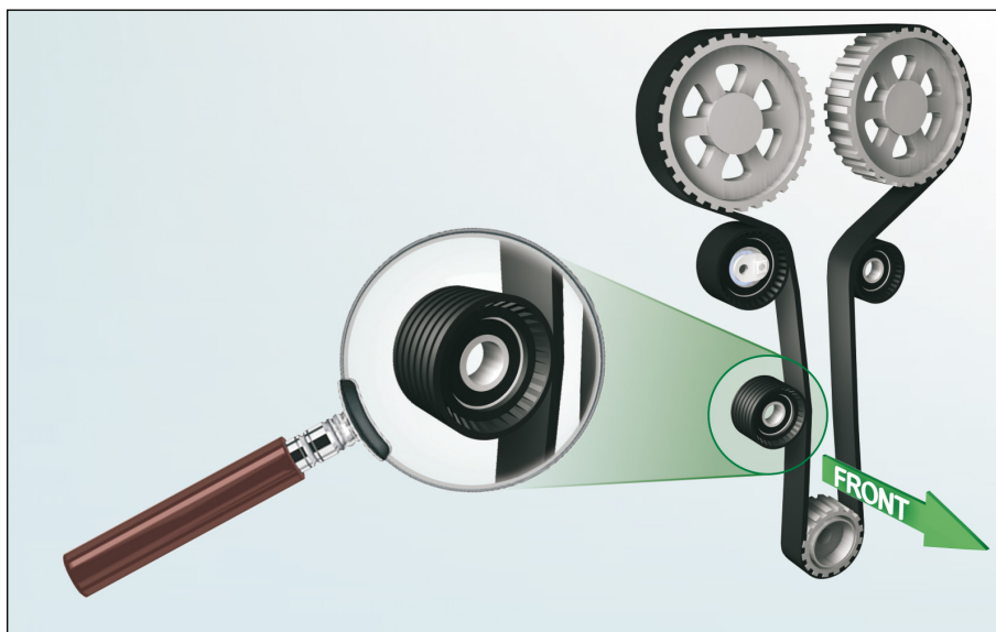
Slika 1: Prihvat remena i pravilan smještaj komponenti u motoru F4R
