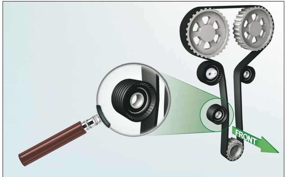
1. ábra: Szíjmenet és görgőpozíció az F4R-motorban
