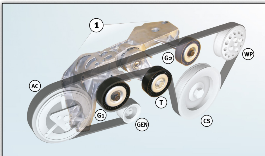
Obrázek 1: 534 0243 10 – nosník s napínací jednotkou v pohonu agregátů a schéma pohonu
