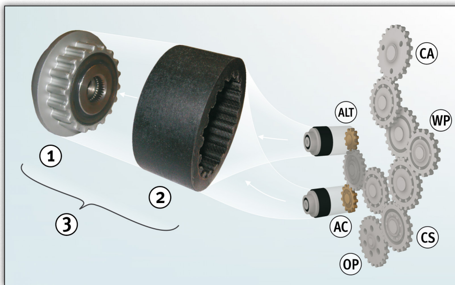
Imagine 1: Rolă cu roată liberă pentru alternator cu manșon de cuplare flexibil și roată dințată cilindrică
