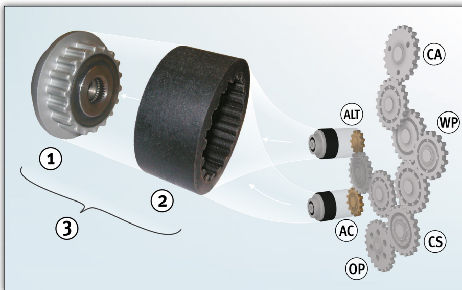
Figur 1: Friløbshjul til generator med en elastisk forbindelsesmuffe og drivsystemet med forreste tandhjul
