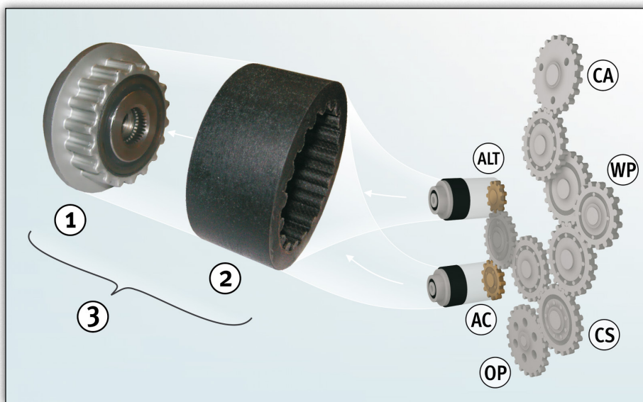
Kuva 1: Laturin vapaapyörä joustavalla liitosholkilla ja sijainnit hammaspyörästössä
