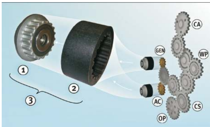
Рис. 1: Шкив генератора с обгонной муфтой, гибкой соединительной муфтой и прямозубым цилиндрическим зубчатым колесом.
