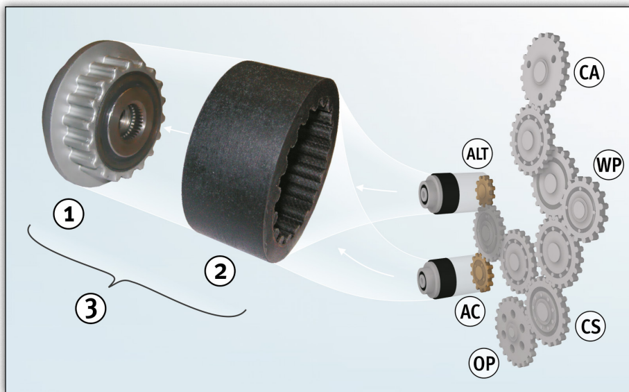
Bild 1: eneratorfrinav med flexibel kopplingsmuff och drivning genom främre kugghjul.
