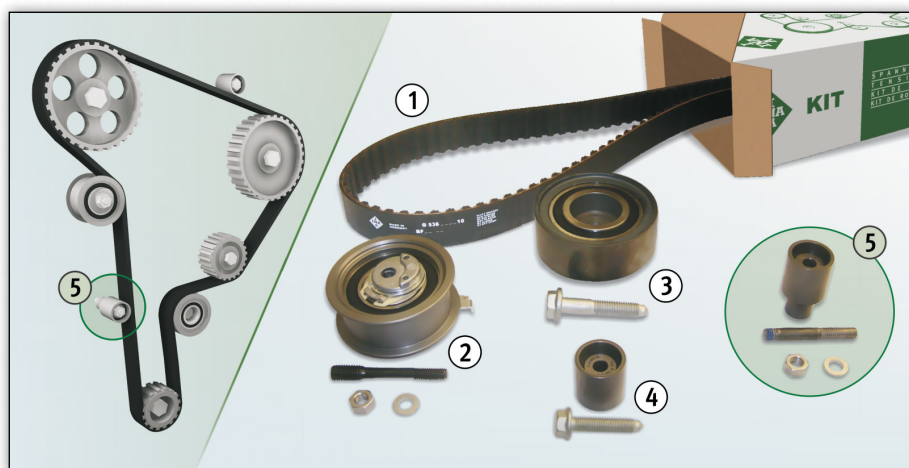
Fig. 1: Diagramă distribuție 1.9 TDI/SDI și conținutul pachetului pentru KIT-urile 530 0361 10/530 0082 10
