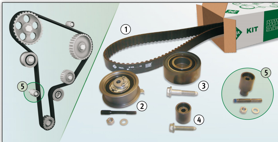
Снимка 1: Диаграма на 1.9 TDI/SDI ремъчно задвижване и съдържание на комплекти 530 0361 10/530 0082 10
