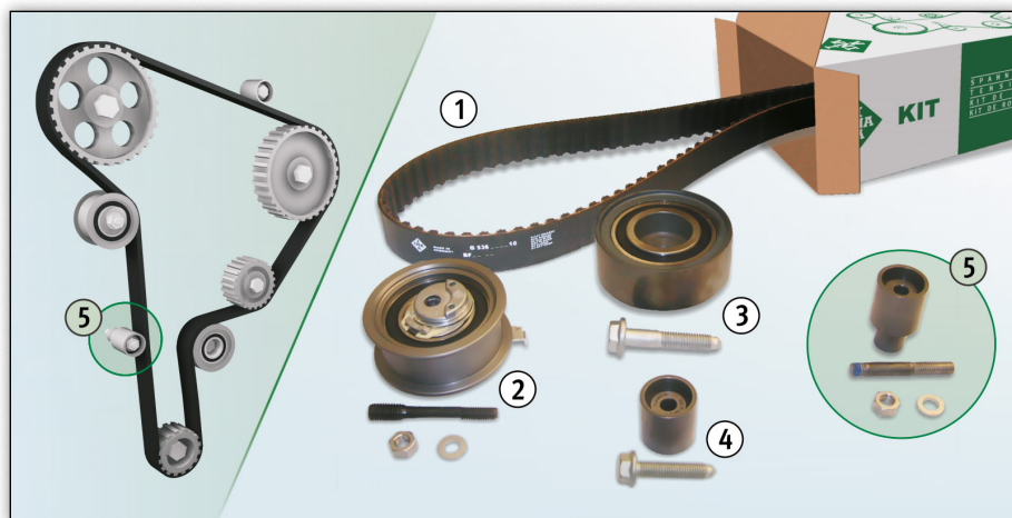
Εικόνα 1: Σχεδιάγραμμα μετάδοσης κίνησης 1.9 TDI/SDI και περιεχόμενα κιτ 530 0361 10/530 0082 10
