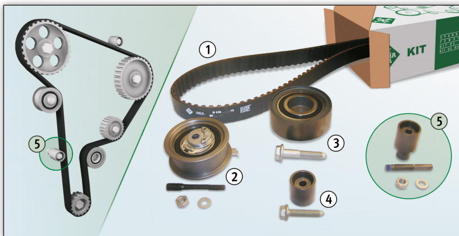
Bild 1: Drivningsschema 1.9 TDI/SDI och innehåll i förpackning KIT 530 0361 10/530 0082 10
