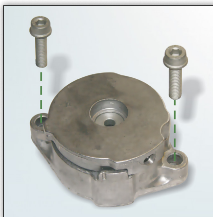
Fig. 1: Design INA cu două șuruburi M8x35
