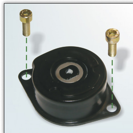
Fig. 2: Design cu două șuruburi M8x22
