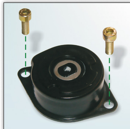
Снимка 2: Модел с два болта M8x22
