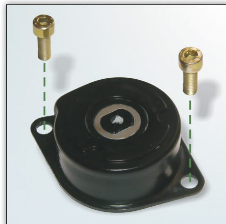
Obrázek 2: Provedení se dvěma šrouby M8x22
