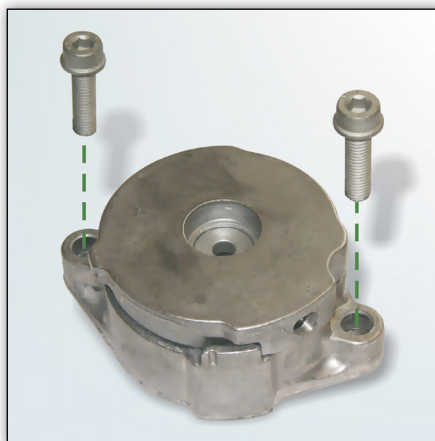
Obrázek 1: INA – provedení se dvěma šrouby M8x35
