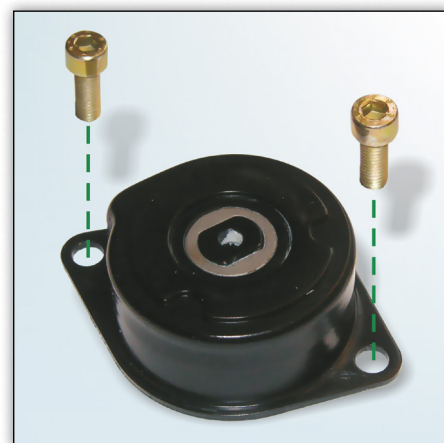
Figur 2: Specifikation med to skruer M8x22
