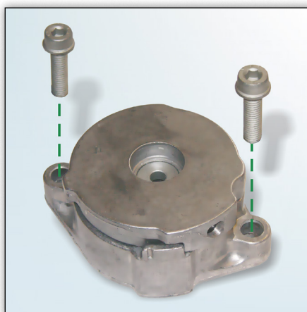
Figur 1: INA – specifikation med to M8x35 skruer
