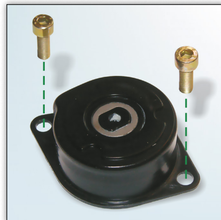
Εικόνα 2: Σχεδιασμός με δύο βίδες M8x22
