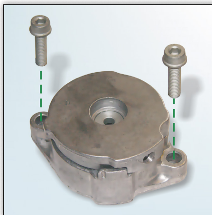
Bild 1: INA – utförande med två skruvar M8x35
