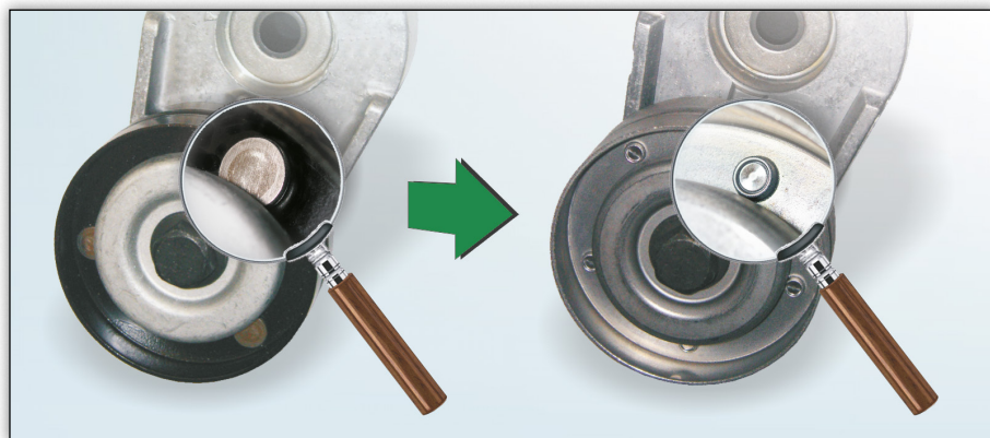
Figur 1: Detaljeret billede af styrerullen i den eksisterende (til venstre) og nye (til højre) udførsel
