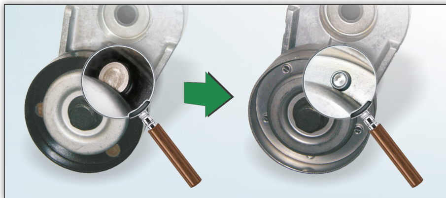
Bild 1: Detaljerad bild på löprulle i tidigare utförande (vänster) och i nytt utförande (höger)
