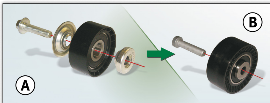
Rolă defletoare 532 0433 10, design precedent (A) și design nou (B).
