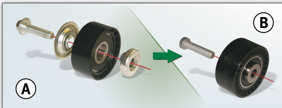
Vodicí kladka 532 0433 10, dosavadní provedení (A) a nové provedení (B)
