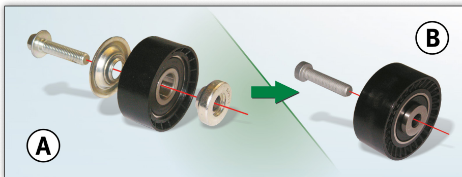
Styrerulle 532 0433 10, eksisterende specifikation (A) og ny specifikation (B)
