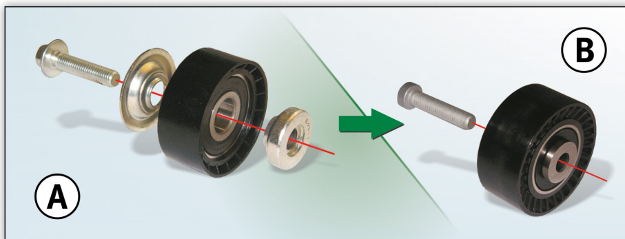
Τροχαλία 532 0433 10, παλαιός (A) και νέος σχεδιασμός (B)
