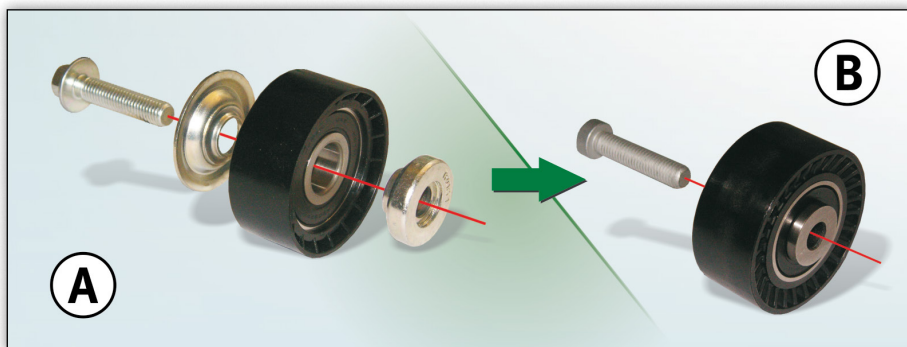
Kuva 1: Ohjainrulla 532 0433 10. (A) Edellinen malli. (B) Uusi malli
