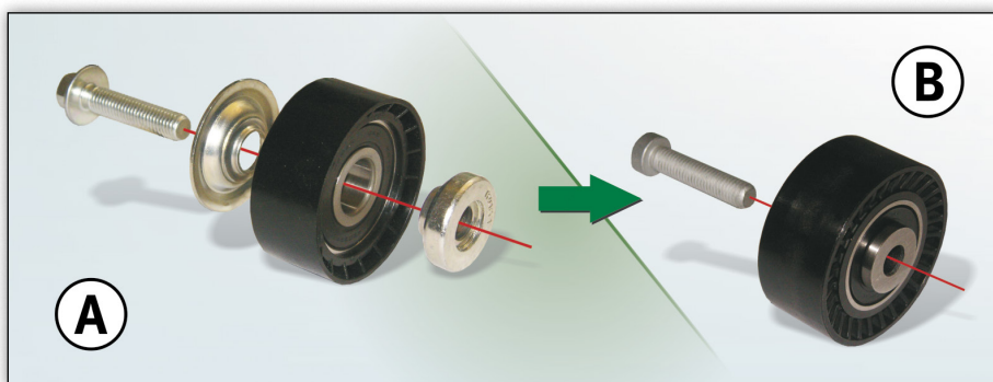
532 0433 10 számú vezetőgörgő, eddigi kivitel (A) és az új kivitel (B)
