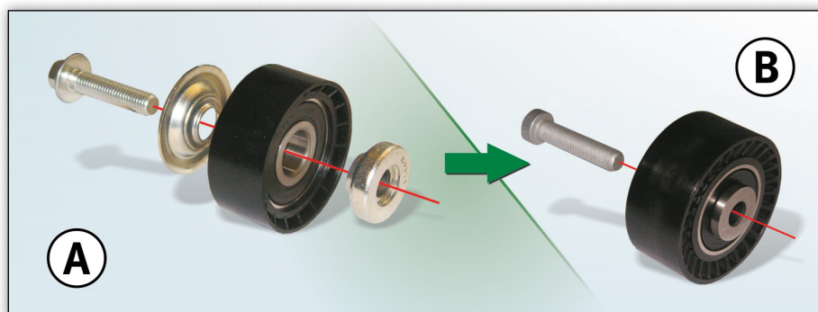
Brytrulle 532 0433 10, tidigare utförande (A) och nytt utförande (B)
