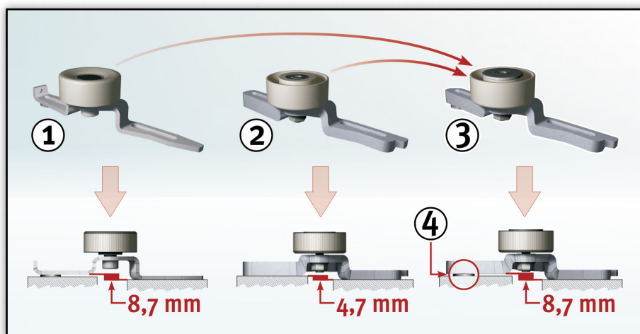
Снимка 1: Илюстрация на отделните обтяжни ролки и техните различия
