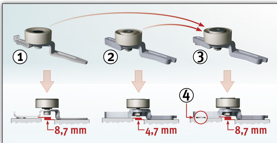
1. ábra: Az egyes feszítőgörgők ábrázolása, azok különbségeivel
