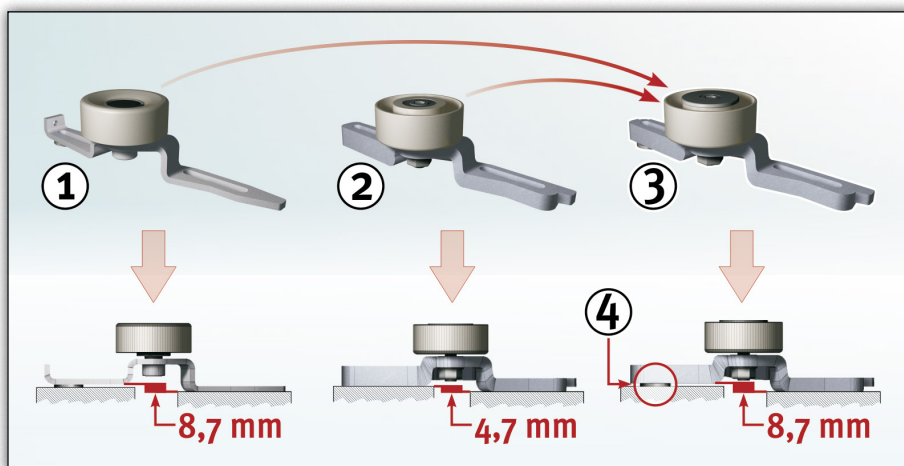
Bild 1: Illustration av de olika spännrullarna och skillnaden mellan dessa
